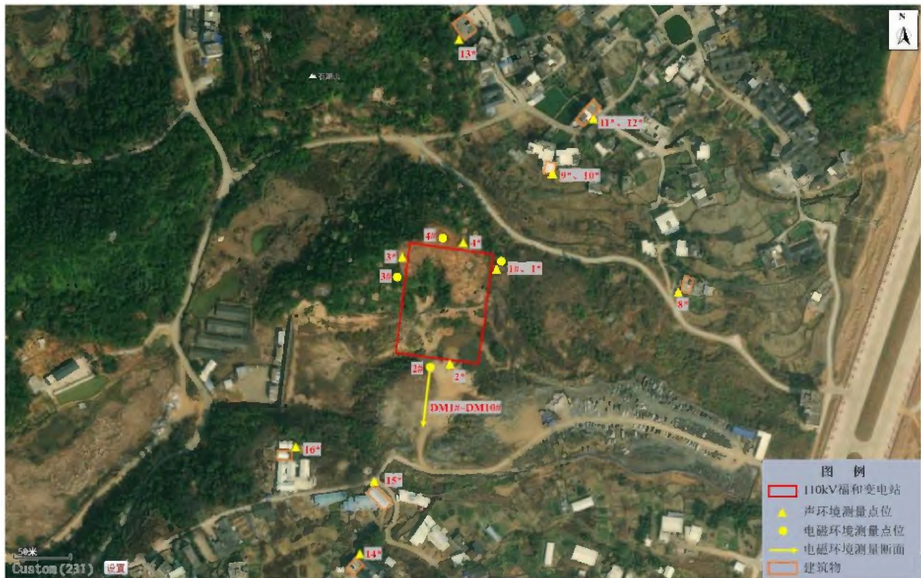
图 I-8-3 河源 110kV 福和站监测布点图
